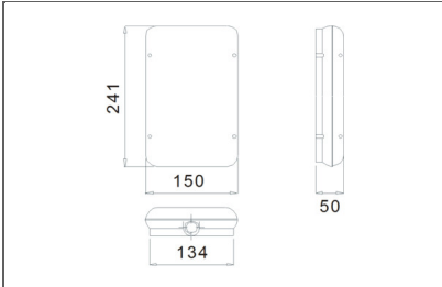
PBS 10
